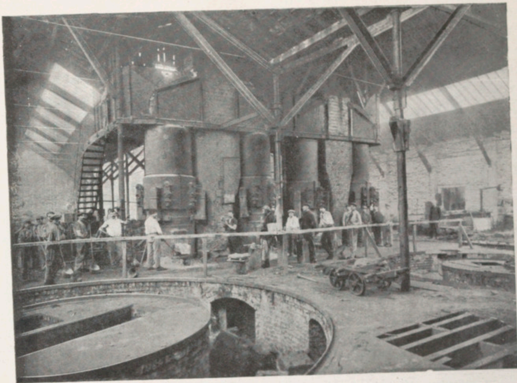
Le groupe de 4 cubilots du " Moulage Mécanique " détruit.
