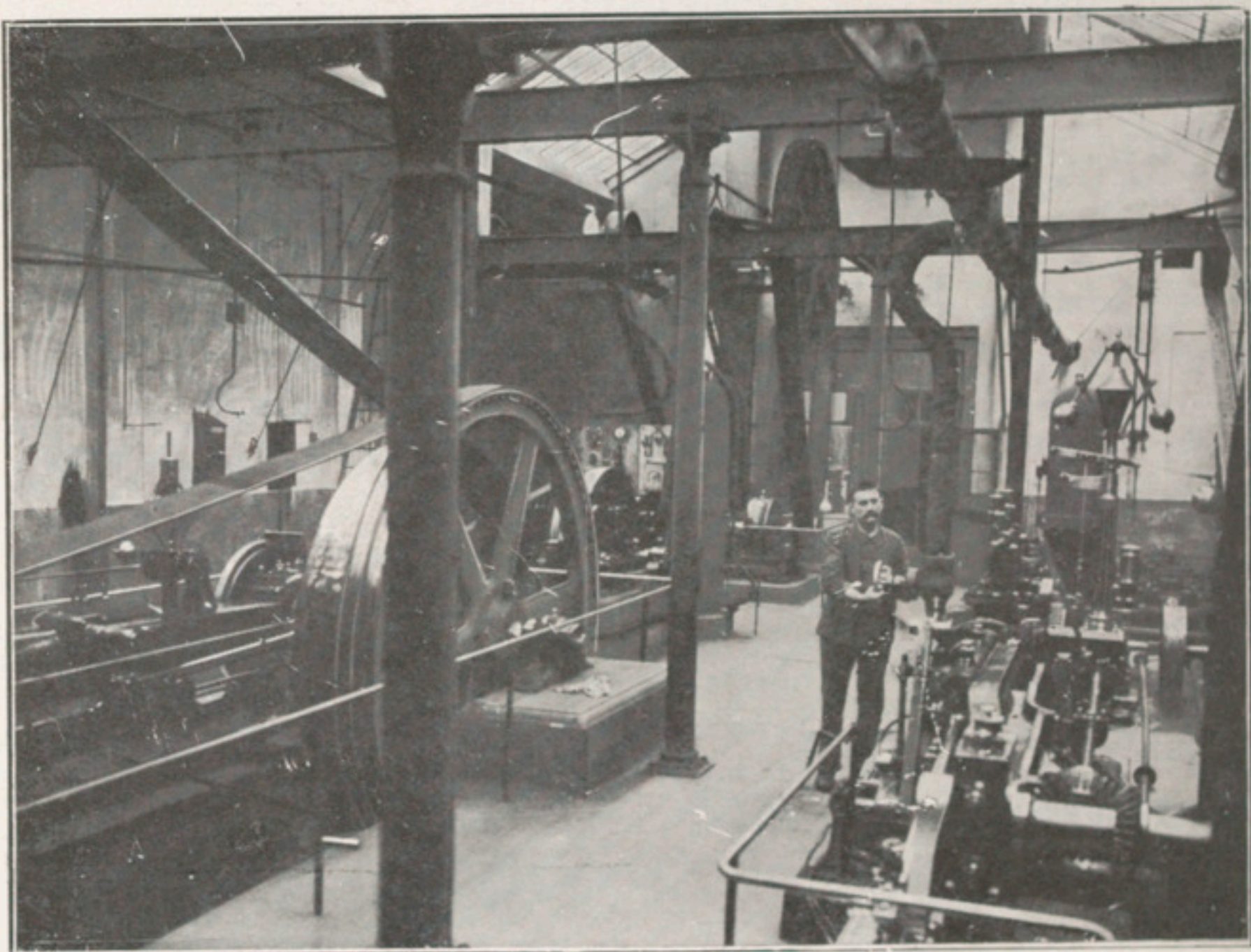
Une salle de machines, à Guise, avant la guerre.
